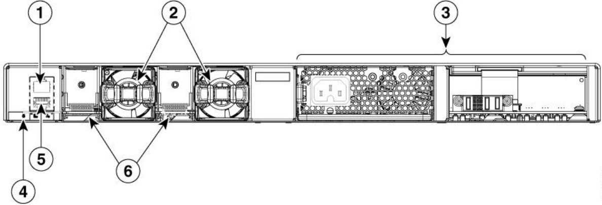
Şekil 6. Bir C9200 Anahtarının Arka Paneli
