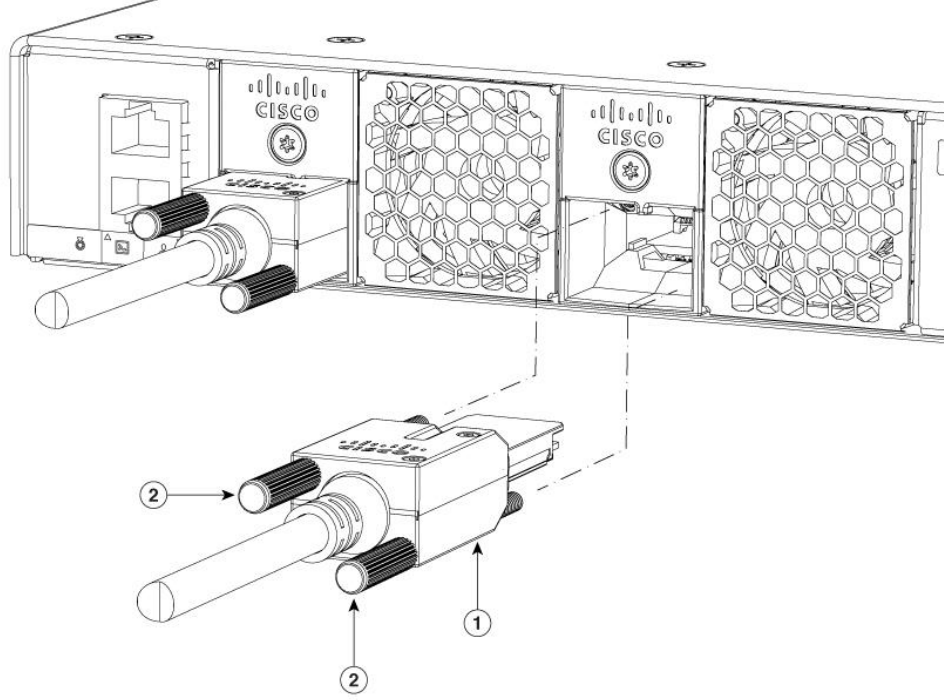
Şekil 13. StackWise Kablosunu StackWise Bağlantı Noktasına Bağlama
