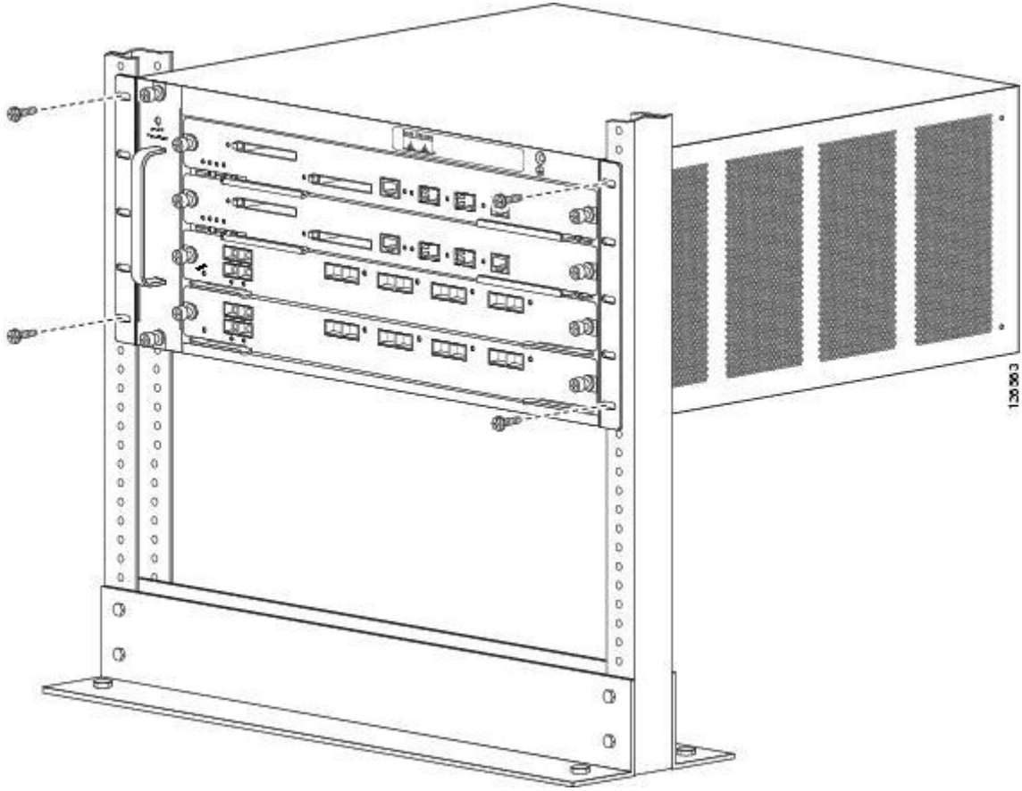
Şekil 1-6 Catalyst 6504-E Anahtar Şasisinin Rafa Takılması
