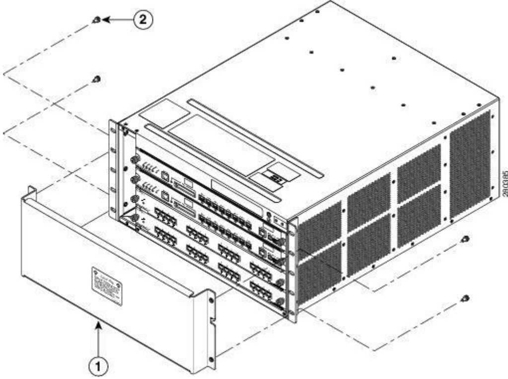
Şekil 1-5 Catalyst 6504-E Kasa Nakliye Braketini Çıkarma
