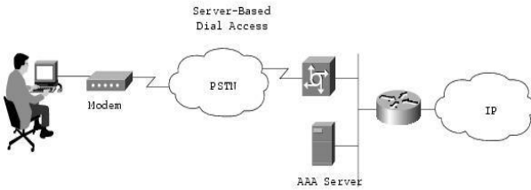
Şekil 1. Küçük LAN Ortamı:
