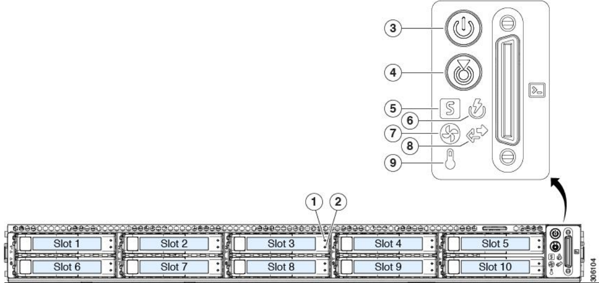
Şekil 1. Ön Panel LED'leri
