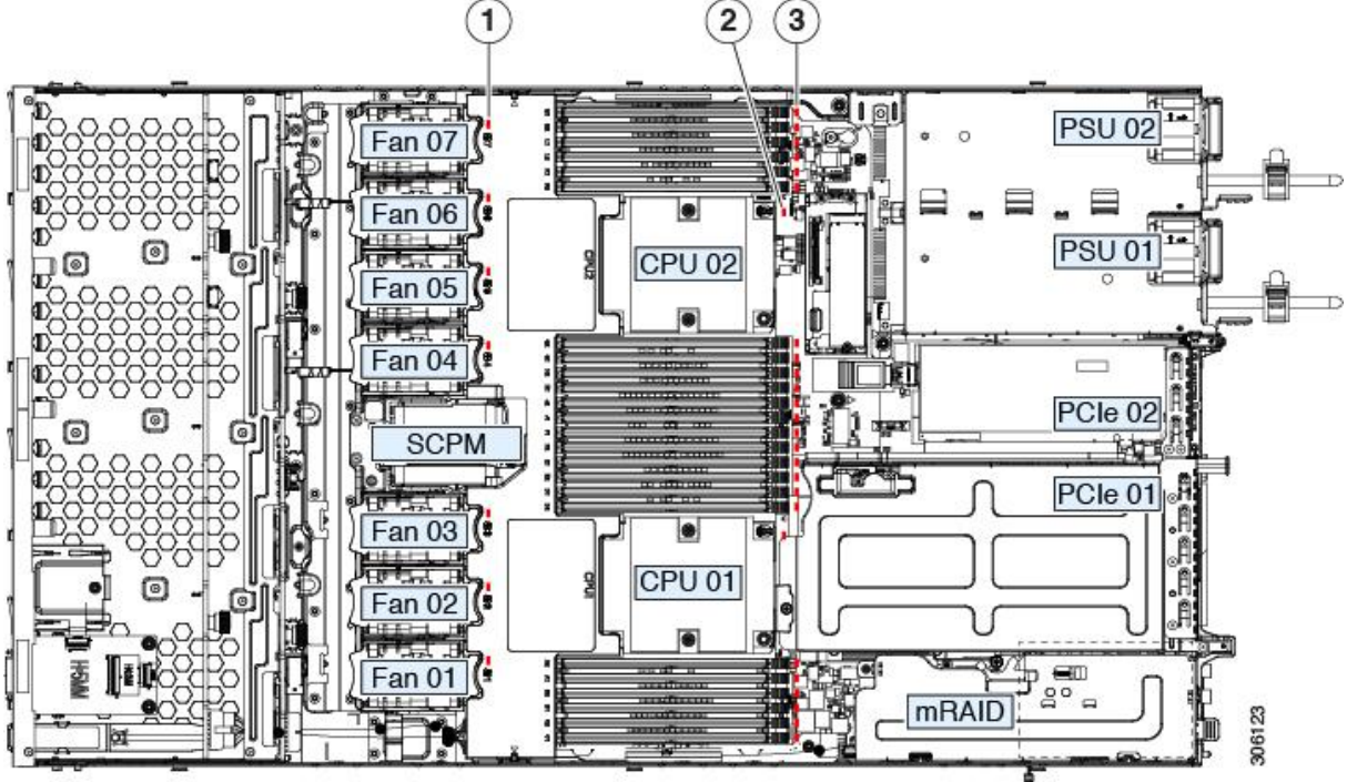
Şekil 3. Dâhili Diyagnostik LED Konumları
