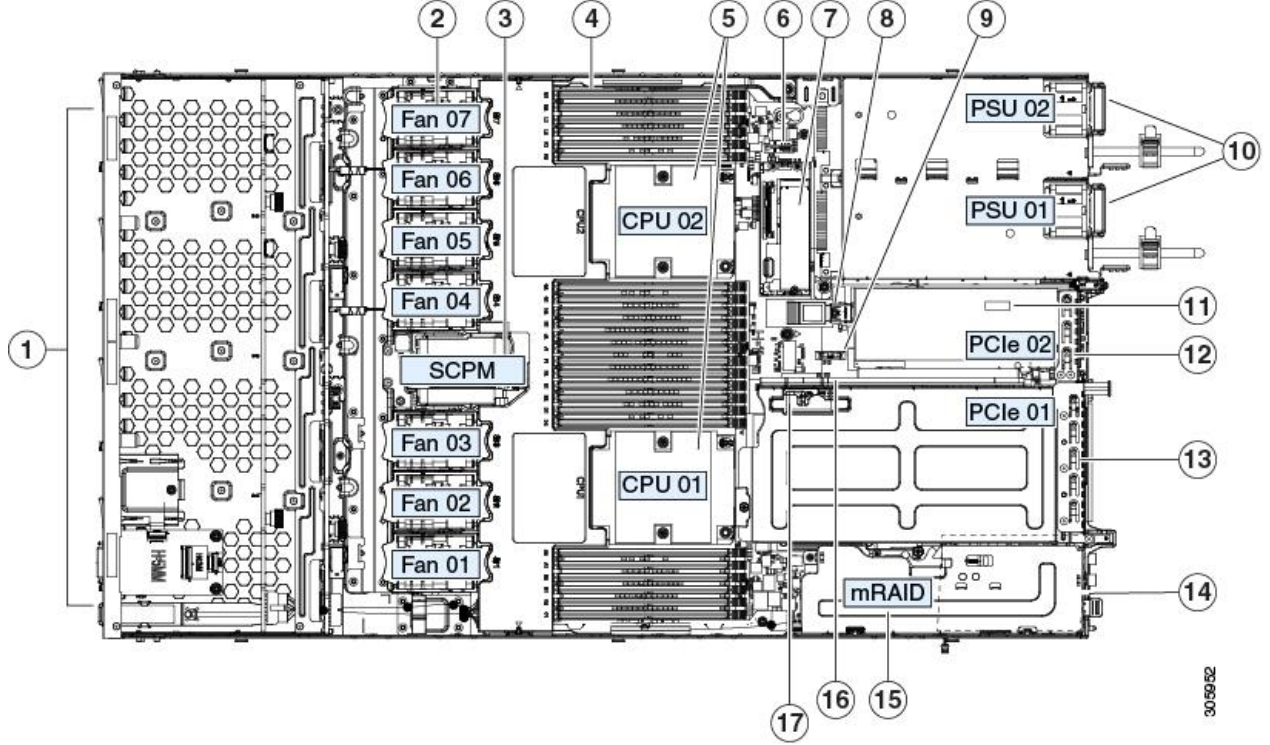
Şekil 4. Cisco UCS C220 M5 Sunucu, Servis Verilebilir Bileşen Konumları
