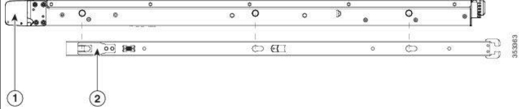
Şekil 1. İç Rayın Sunucu Tarafına Takılması
