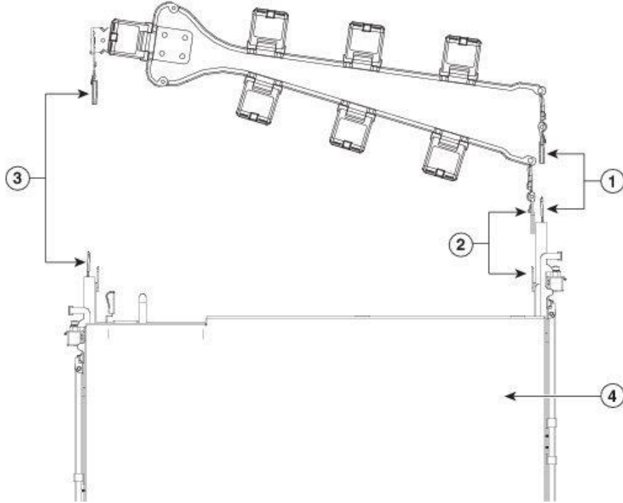
Şekil 4. CMA'nın Kayar Rayların Arka Uçlarına Takılması
