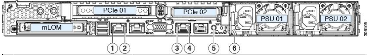
Şekil 2. Arka Panel LED'leri
